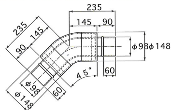
ST管
