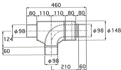
NT管
