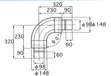
STR管
