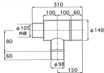
NT管
