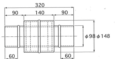
ニップル
